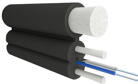
Рисунок 1 - Общий вид
