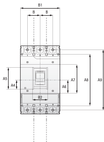
Рис.1 Габаритные размеры AV POWER-1 (2) (3) (4)
