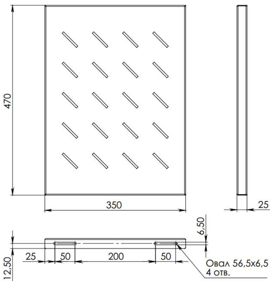
Рисунок 2 - Габаритные размеры
