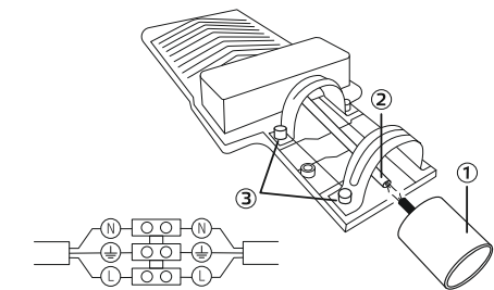
Рис. 1. Монтаж светильника
