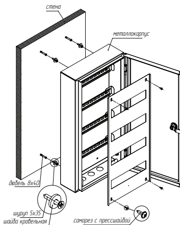
Рис. 1.1 Схема настенного монтажа
